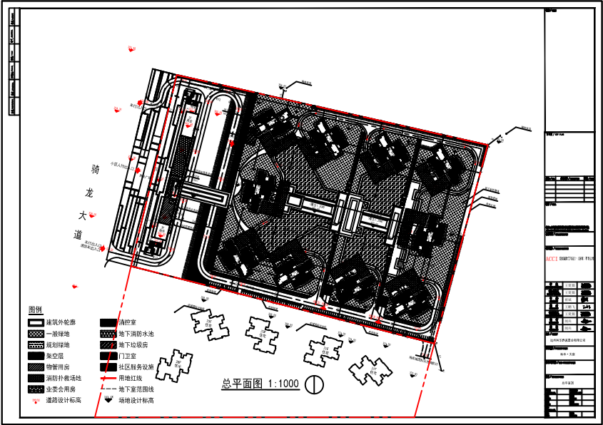
科华·天宸项目规划审批总平面布置图
