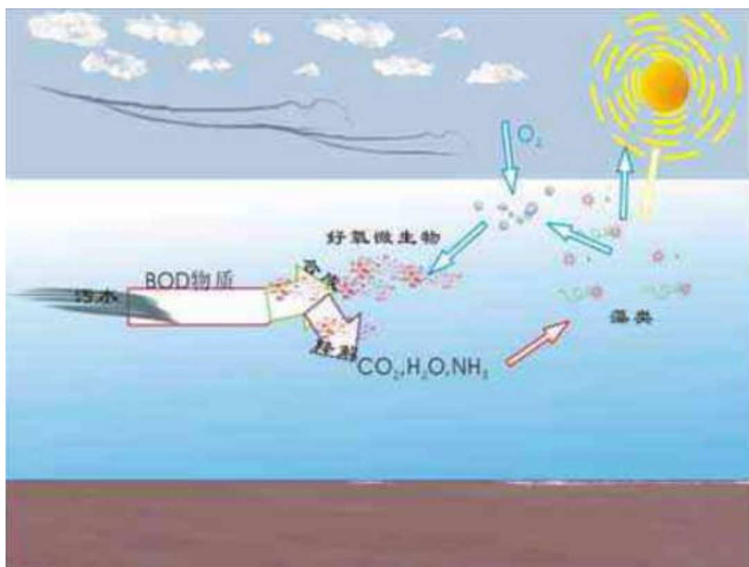
图 4-8 好氧塘工作原理图
