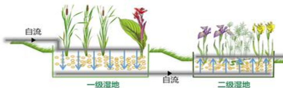
图 4-5 二级人工湿地示意图
