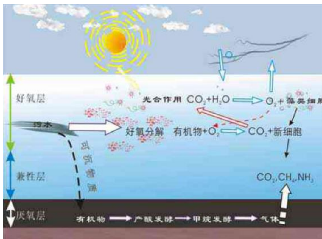
图 4-9 兼性塘工作原理图
