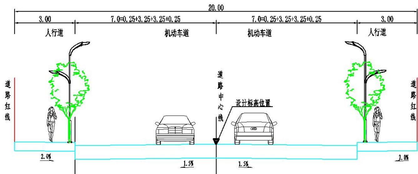
道路标准横断面图
