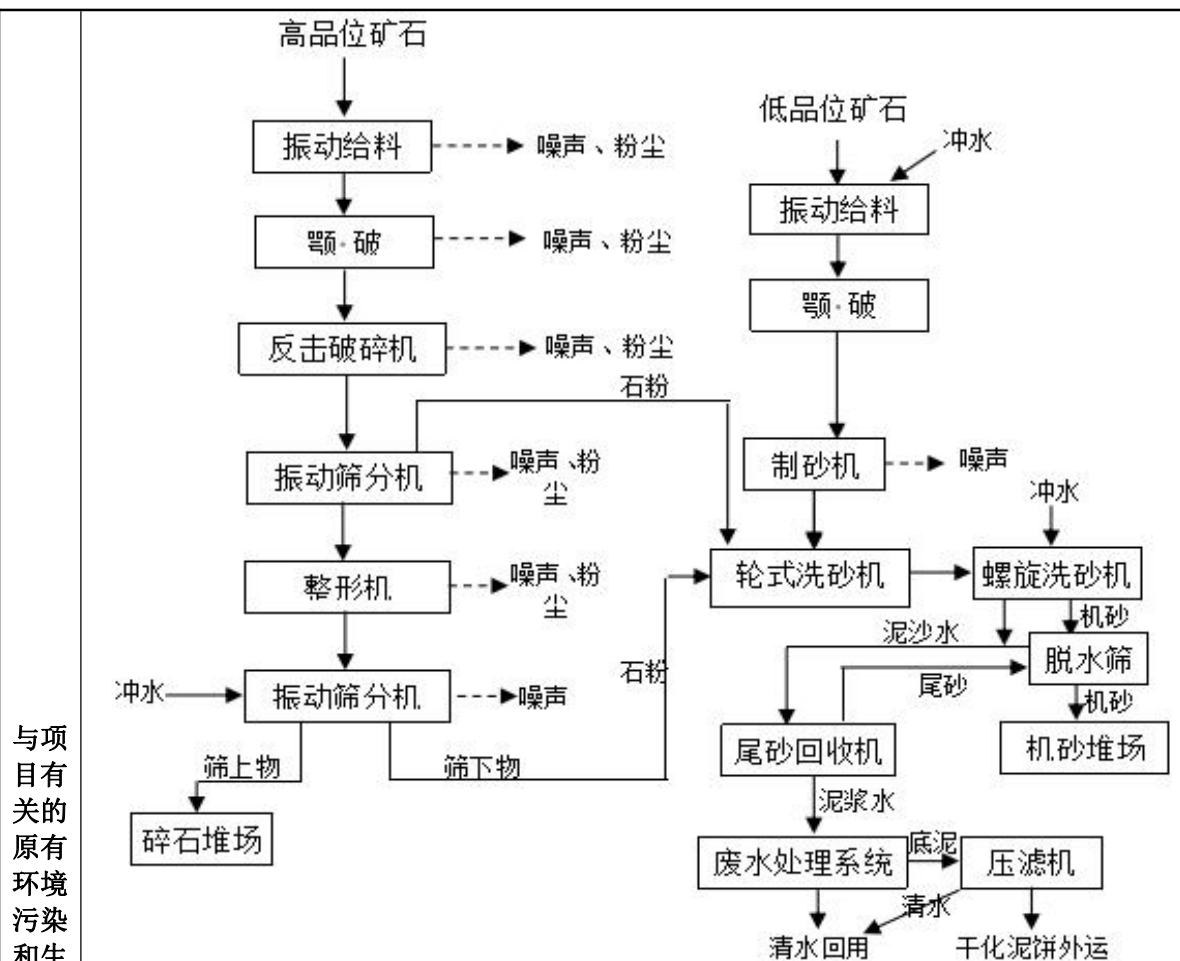
图17: 原工程加工区生产工艺流程及产污环节图
