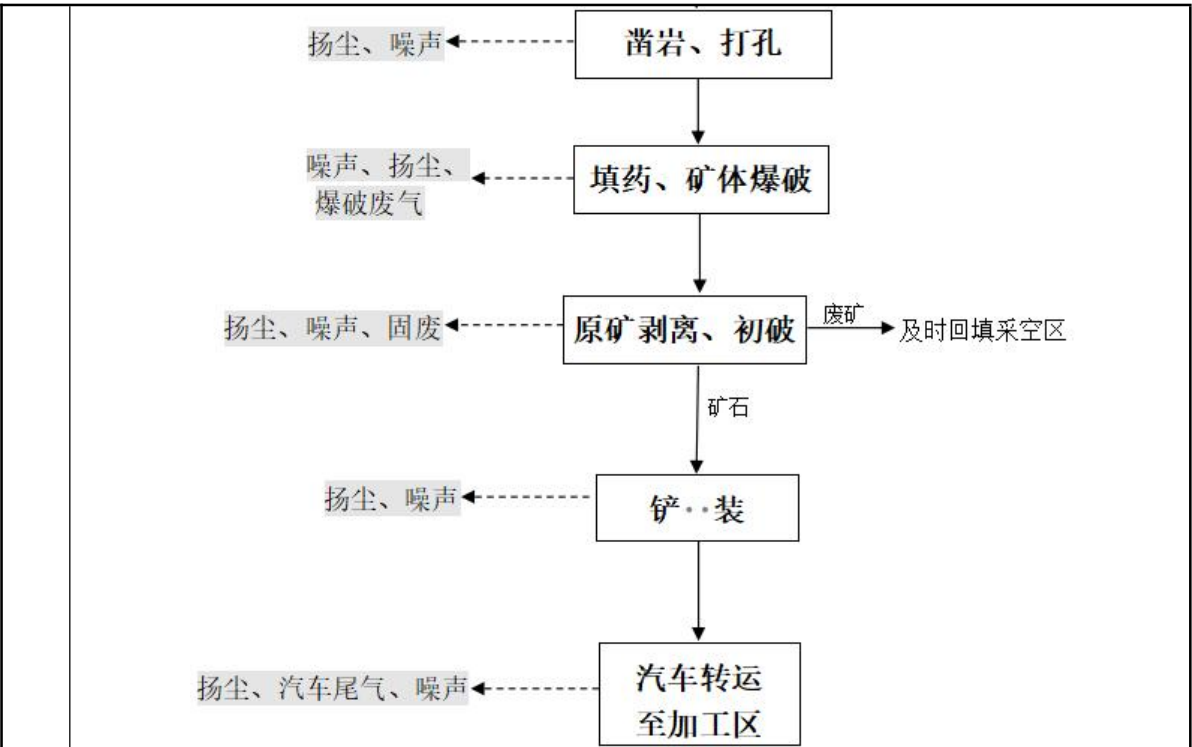
图11：矿山开采工艺流程及产污环节图
