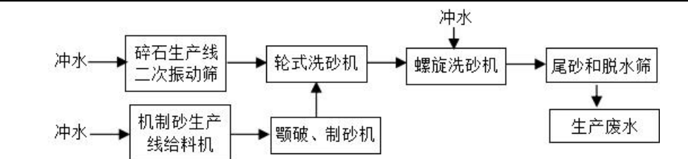
图20：生产废水产生及流向示意图
