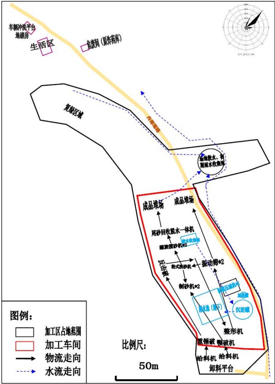
图9：项目加工区平面布置图
