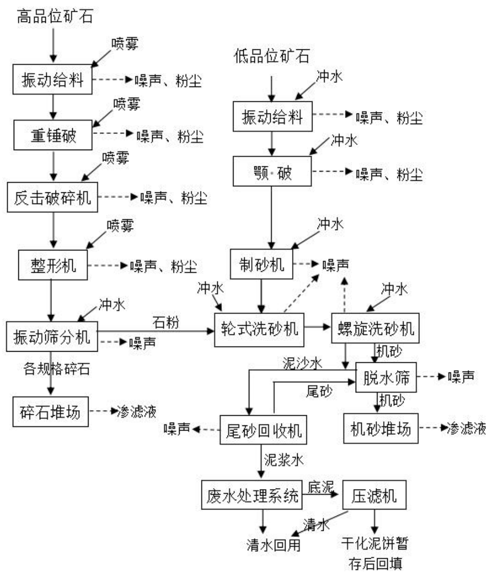
图13：运营期加工工艺流程及产污环节图
