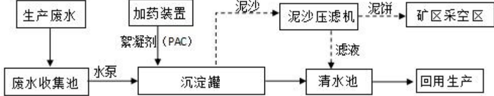
图21：生产废水处理工艺流程图
